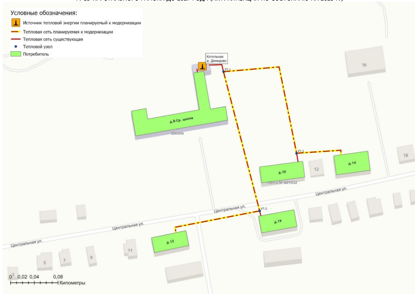
Рисунок 4.1.1 - Сценарий перспективного развития системы централизованного теплоснабжения котельной д. Демидово (до момента газификации населенного пункта)
