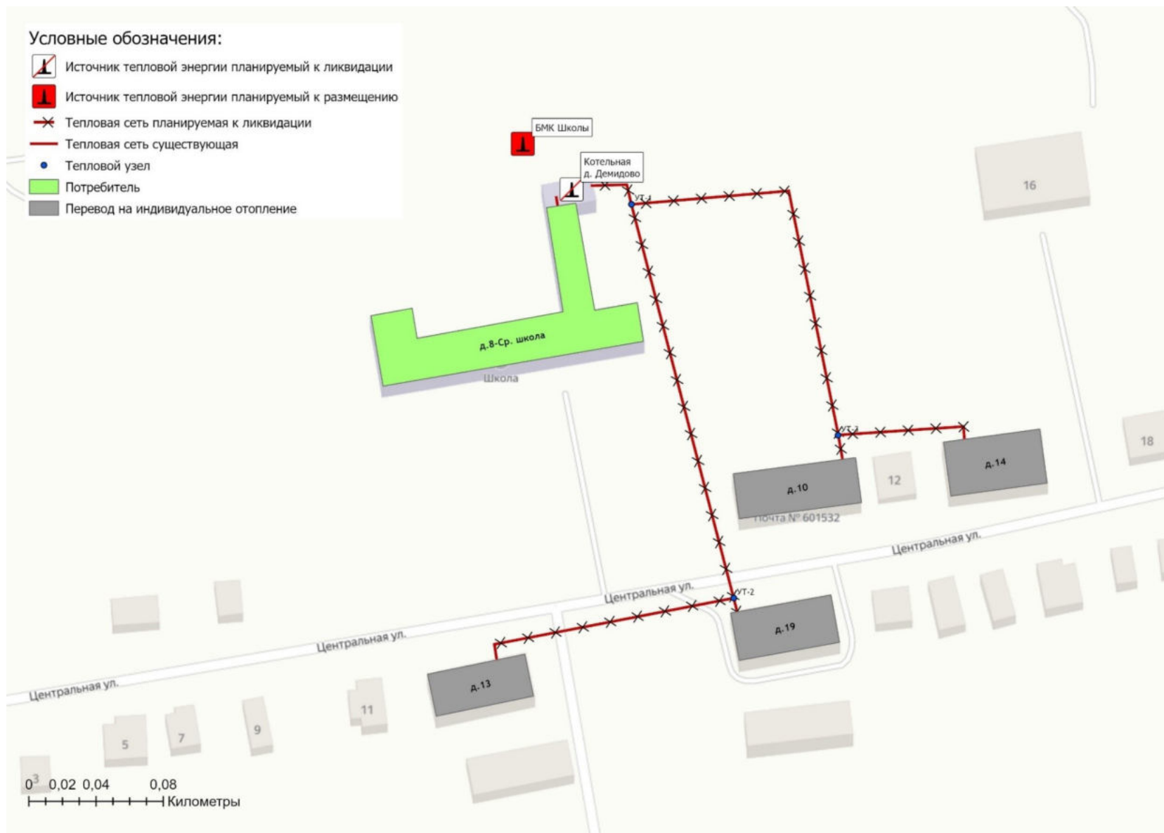
Рисунок 4.1.2 - Сценарий перспективного развития системы централизованного теплоснабжения котельной д. Демидово (после газификации населенного пункта)
