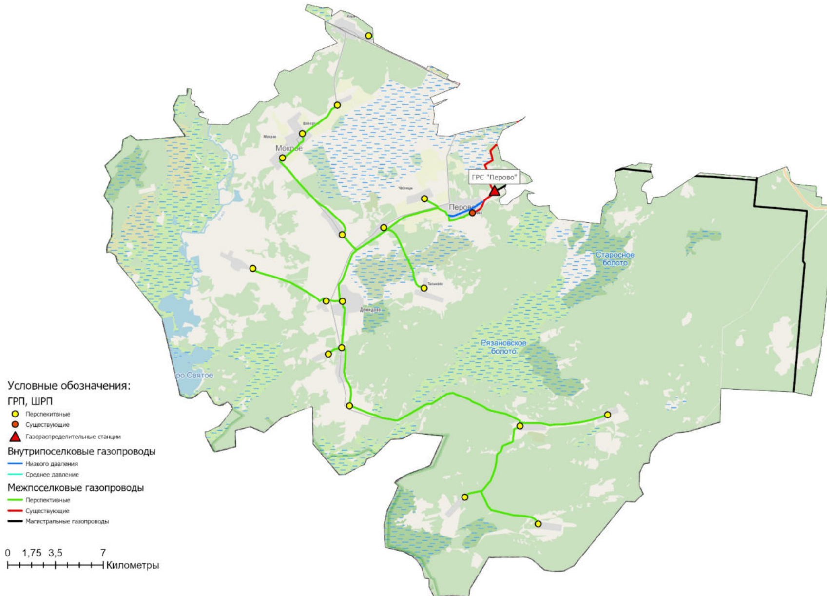
Рисунок 8.5.1 - Перспективная схема газификации муниципального образования Демидовское (сельское поселение)
