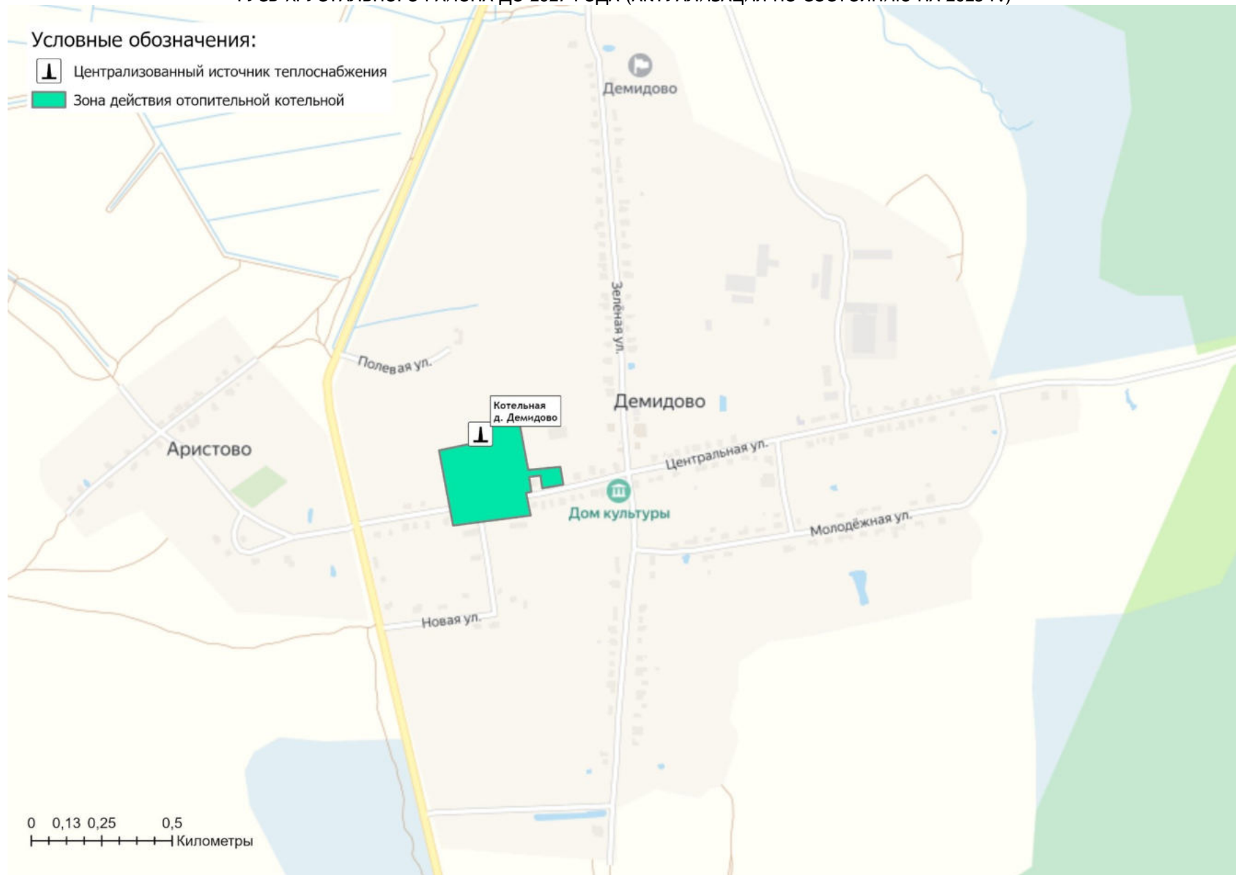
Рисунок 1.4.1 - Зона действия отопительной котельной на территории муниципального образования Демидовское (сельское поселение)
